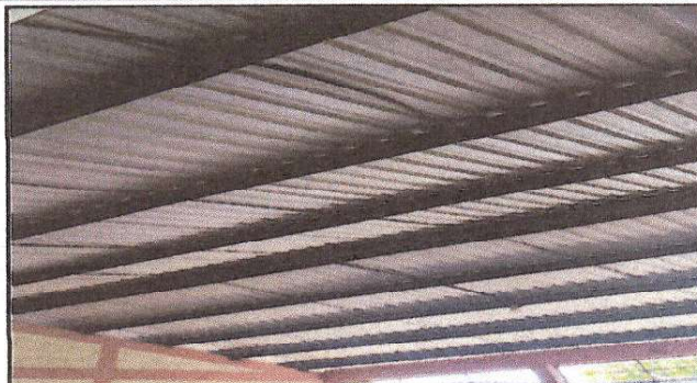
Foto 2: Sustitución de lámina, por lámina troquelada aluzinc calibre 26 Sustitución de capote de lámina para lámina acanalada Sustitución de elementos de fijación
